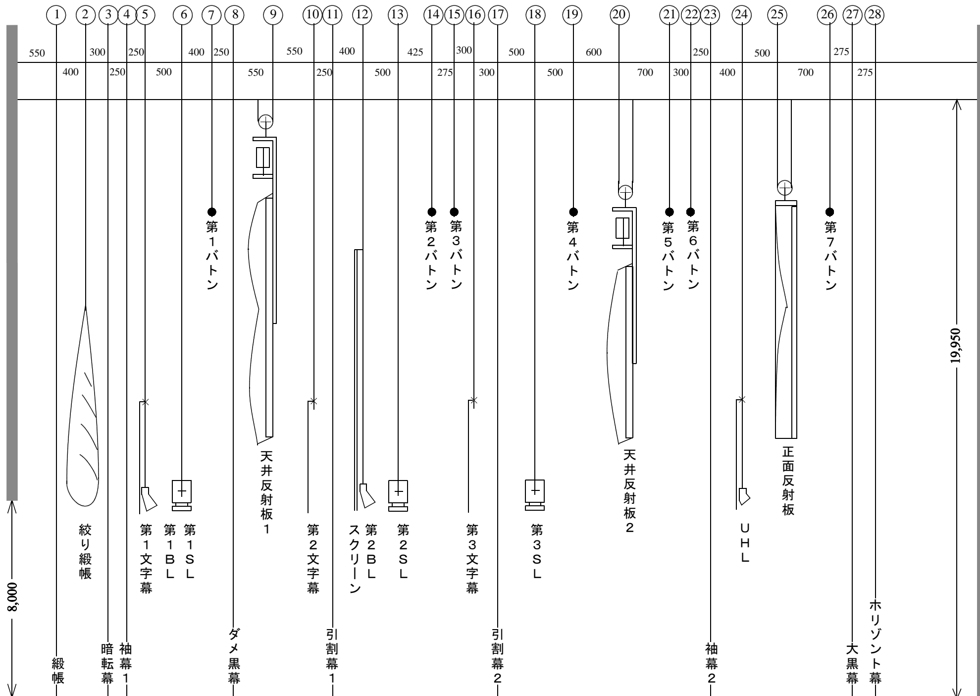
さつきホール吊り物配列図
